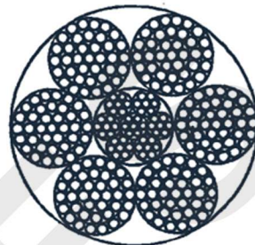
6 x 37 + IWRC
